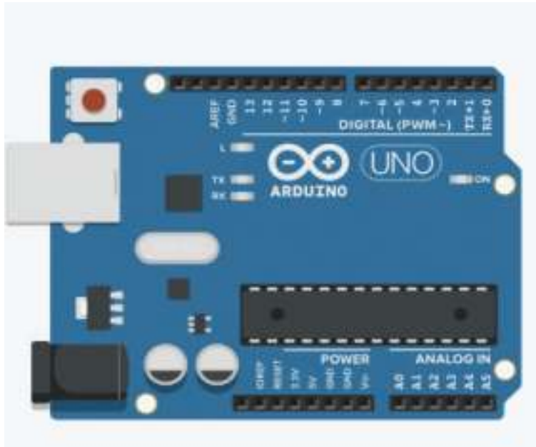
Gambar 9.2 Pin Arduino Uno
