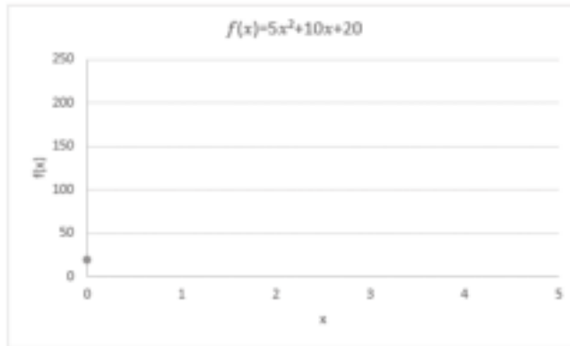
Gambar 7.6 Tampilan Grafik f(x)
